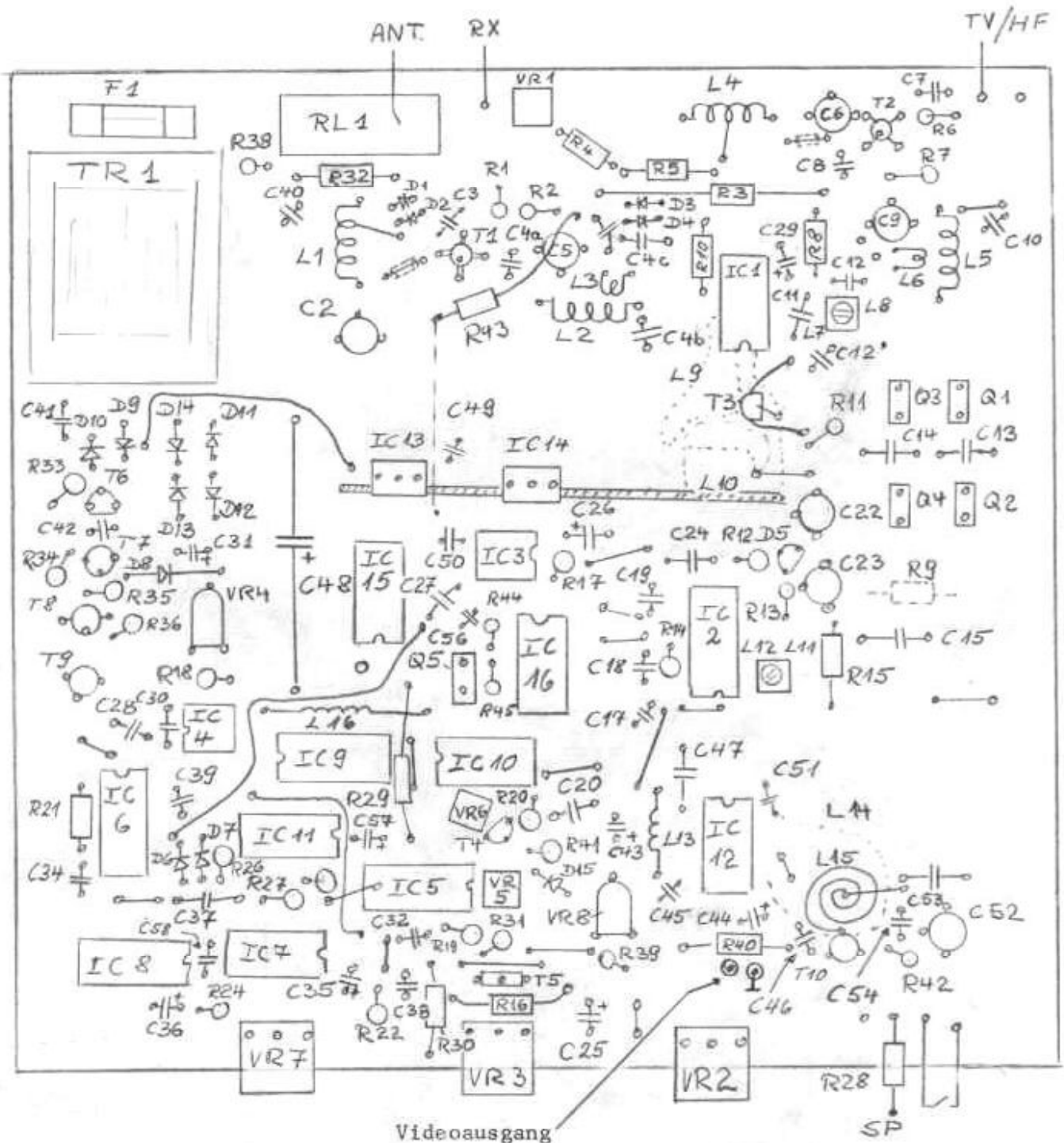
Panorama-Empfänger PC-220, Bestückungsplan
