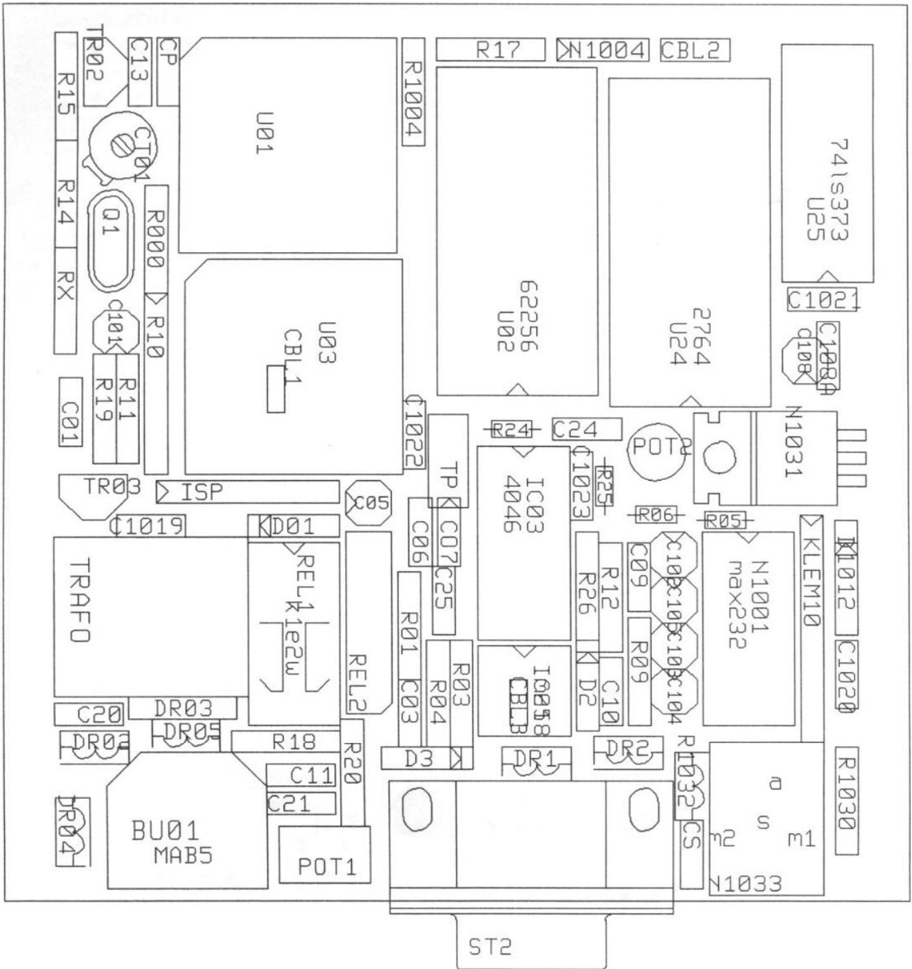
SC-4 WRAASE electronic Bestückungsplan
